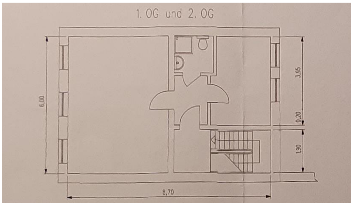
Wohnzimmer mit Küche, Schlafzimmer, Diele, Bad 39 qm im 1. und 2. OG
